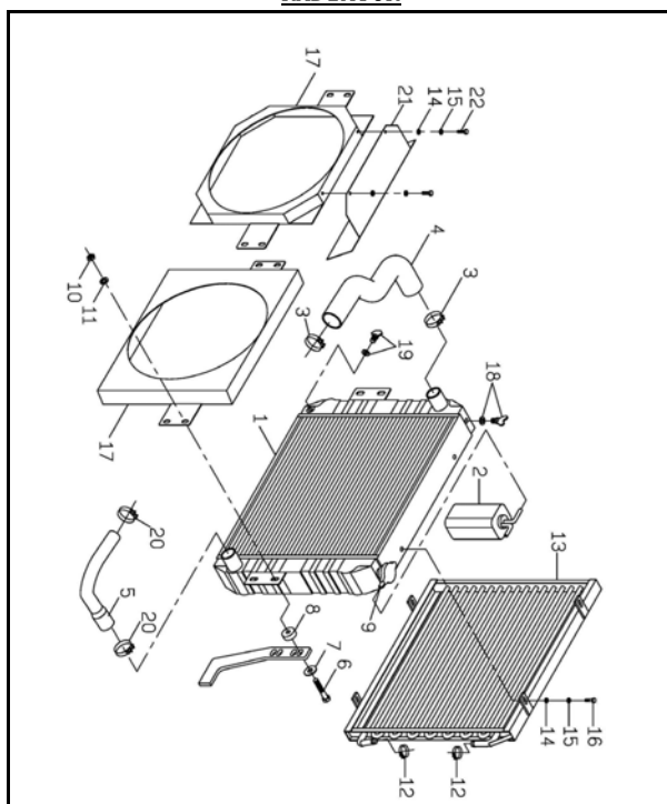
散热器組 A304-2A GM3.0 RADIATOR
