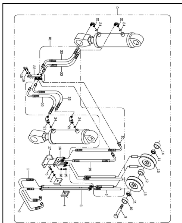
二截式傾卸配管組
