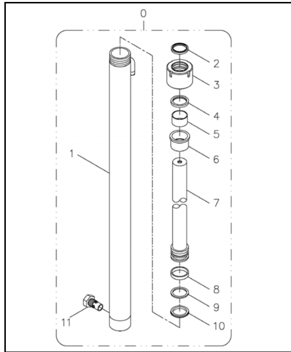
二. 三截式升降缸組 (左)
