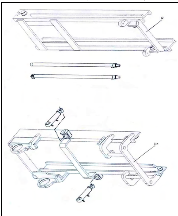
滑軌組 A308-2A MAST ASSY
