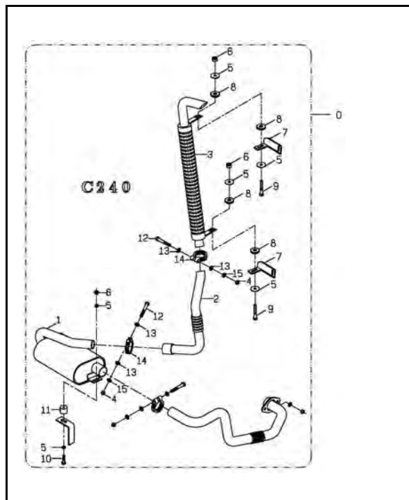
向上排氣管組
