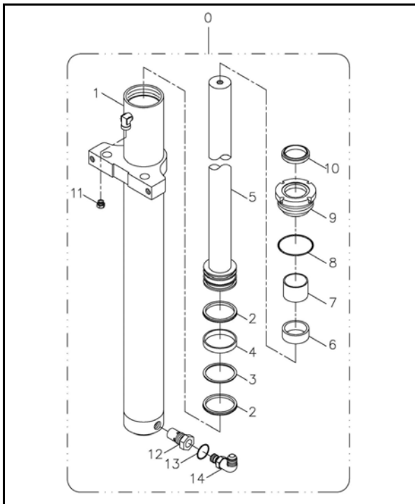
二. 三截式貨櫃型油壓缸組
