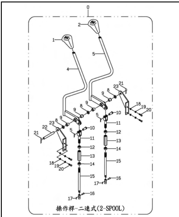
操作桿組 A307-2 LINKAGE LEVER ASSY
