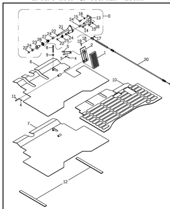
加速器連桿組 A305-4 ACCELERATOR LINK
