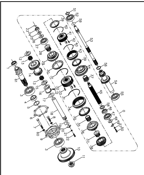
手排傳動齒輪組 A301-3 (MT) TRANSMISSION GEAR SET
