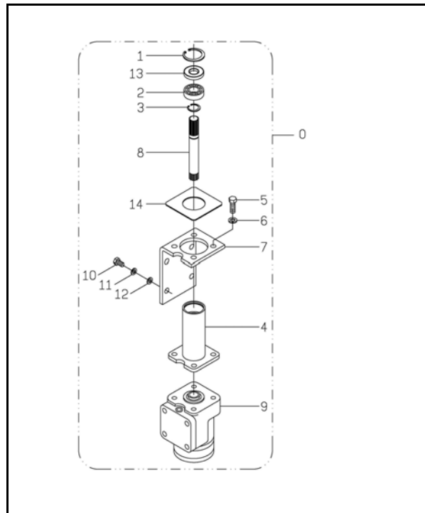
油壓方向機 A303-4 POWER STEERING
