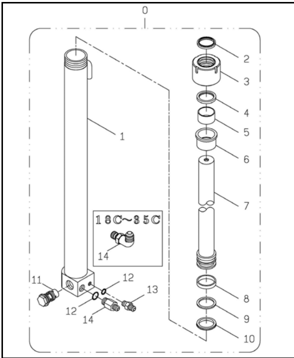
二. 三截式升降缸組 (右)
