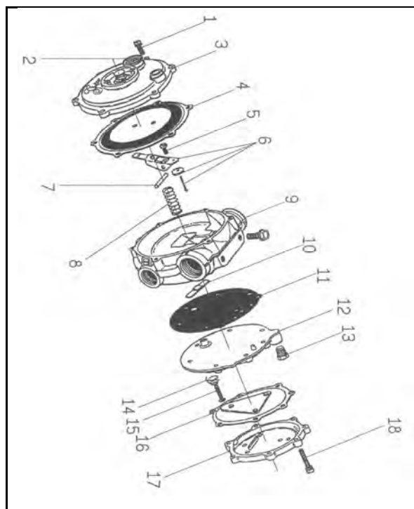
轉換器 A311-2 LPG CONVERTER
