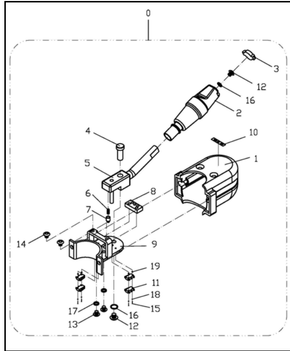
電子式自排排檔開關組 A307-1A (AT)ELECTRIC SHIFTLEVER SWITCH
