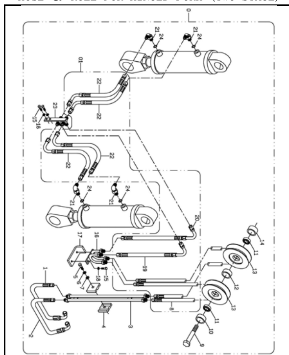
三截式傾卸配管組
