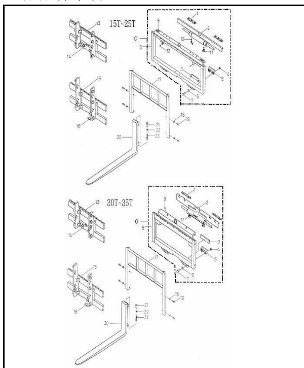
側移組 A310-1 SIDE SHIFT
