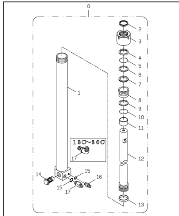
二截式貨櫃型升降缸組 (右)
