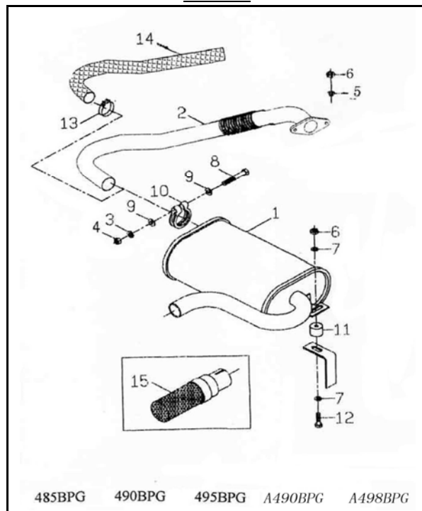
消音器組 A304-3B EXHAUST
