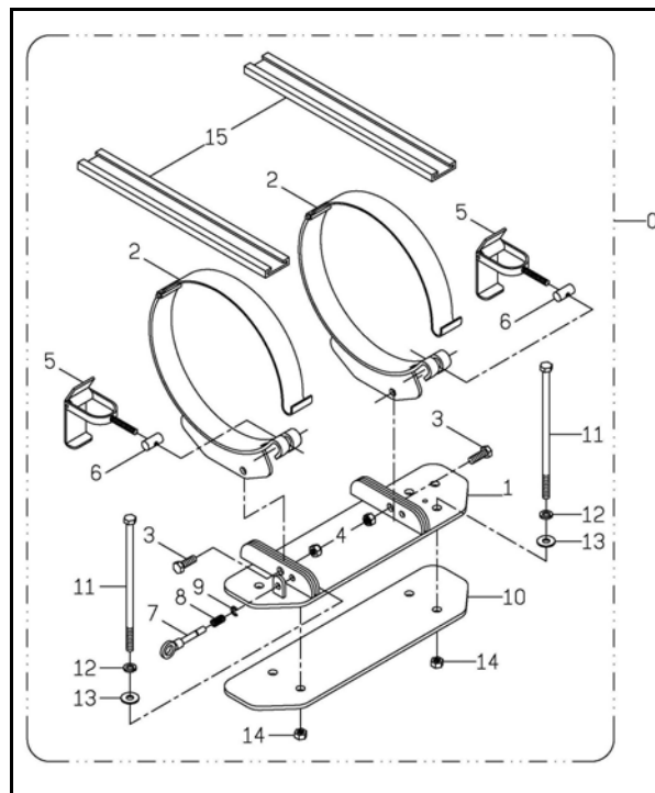
立式瓦斯桶架
