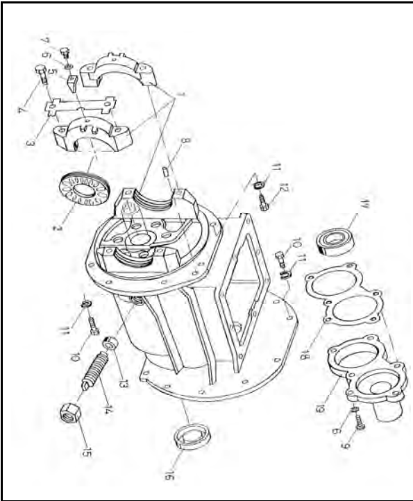
手排變速箱組 A301-1 (MT) TRANSMISSION
